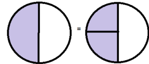
\frac{1}{2}
